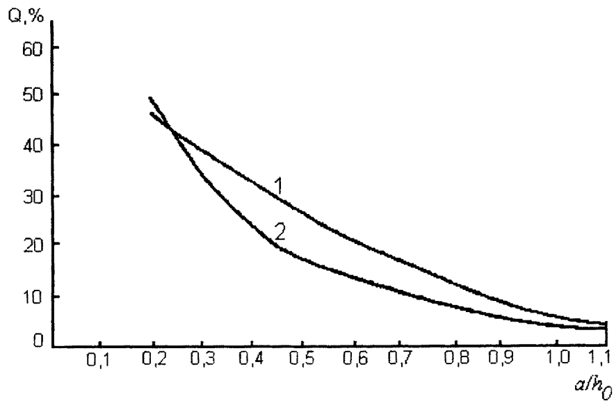
Рис. ПЗ.3. Зависимость доли перелившейся через обвалование жидкости Q от параметра a/h : 1 - расчет; 2 - эксперимент
