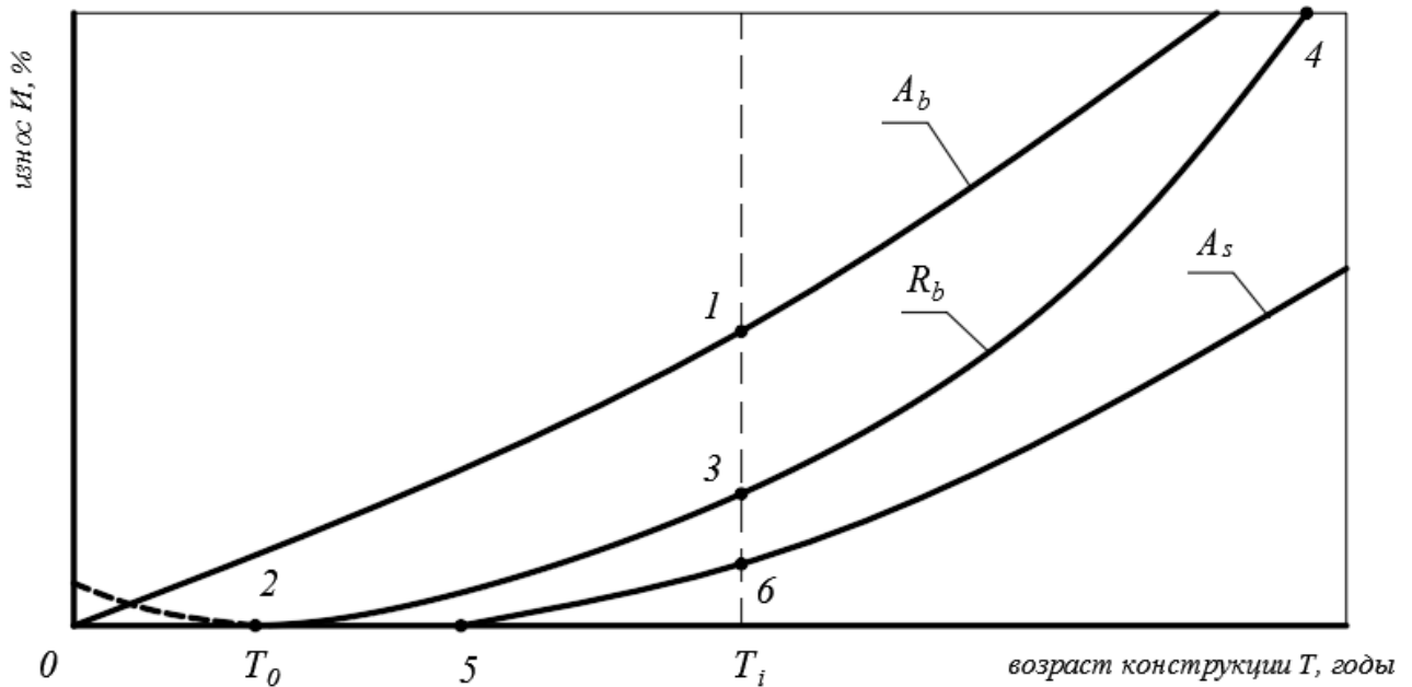
Рисунок В.3 – Изменение во времени поперечного сечения конструкции A_b , прочности ее бетона R_b и площади арматуры A_s из-за коррозии: 1 – фактическая площадь бетона на момент идентификации; 2 – прочность бетона на момент T_0 ; 3 – уменьшенная прочность бетона на момент идентификации; 4 – предельное снижение прочности бетона (предельный износ); 5 – продолжительность карбонизации защитного слоя бетона; 6 – зафиксированный процент коррозии на момент идентификации
