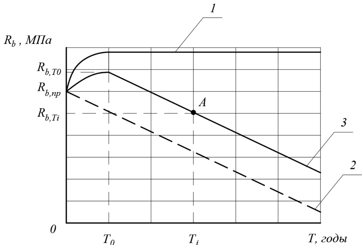
Рисунок В.1 – График изменения прочности бетона конструкции: 1 – кривая роста прочности; 2 – кривая деградации; 3 – итоговая теоретическая кривая изменения прочности
