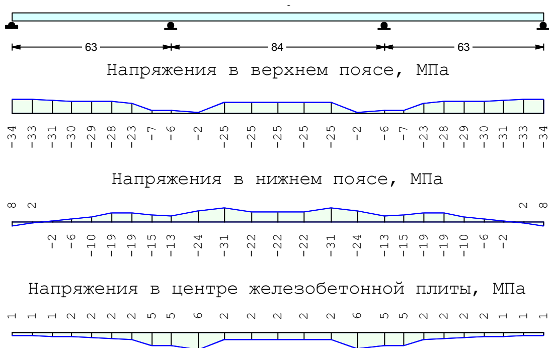
Рисунок 9 – Эпюры напряжений от воздействия усадки бетона
