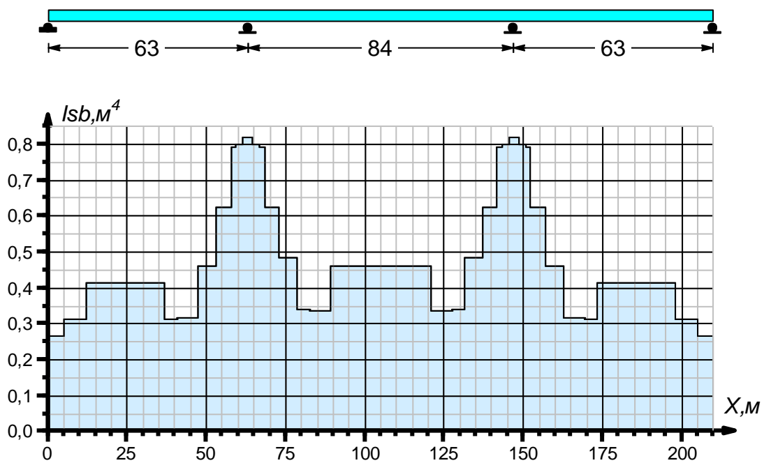
Рисунок А.6 – Эпюра моментов инерции сталежелезобетонной балки
